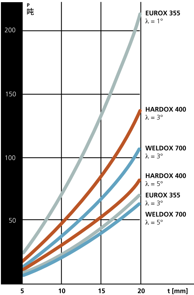
图3 剪切与钢板厚度及刀面角λ之间的关系
